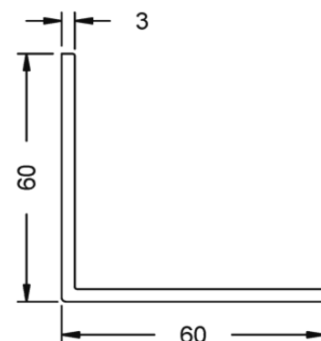
18784 - Profilo angolare da 60/60/3 mm.
