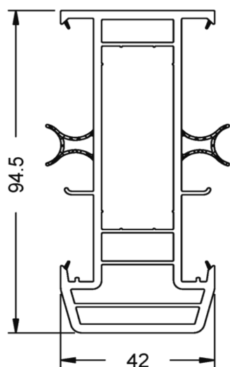
19211 - Profilo Lesena 94,5/42 Classic 70
