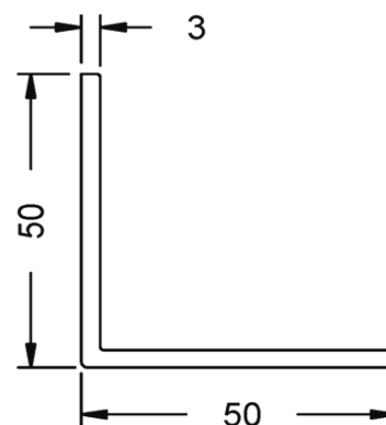
17170 - Profilo angolare da 50/50/3 mm.
