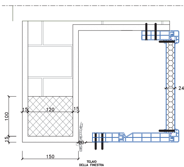
Versione standard da 24 mm.
