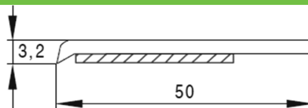
67050 - Piatta con biadesivo da 50 x 3 mm.
