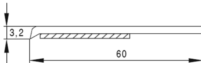
67060 - Piatta con biadesivo da 60 x 3 mm.
