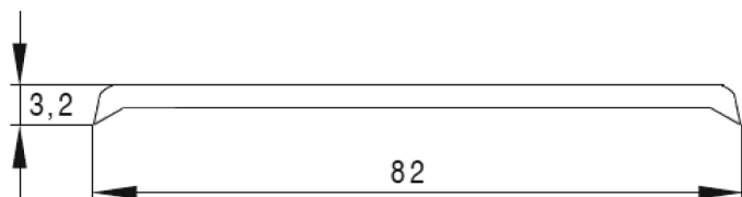
67S82 - Piatta senza biadesivo da 82 x 3 mm.
