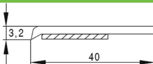
67040 - Piatta con biadesivo da 40 x 3 mm.
