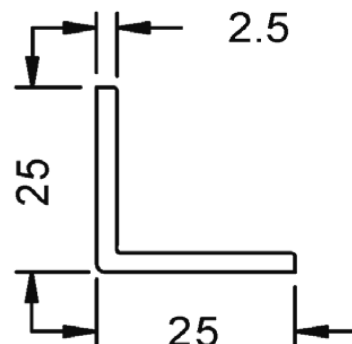
19306 - Profilo angolare da 25/25/2,5 mm.
