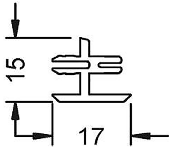
18423 - Profilo di accoppiamento 15/17
