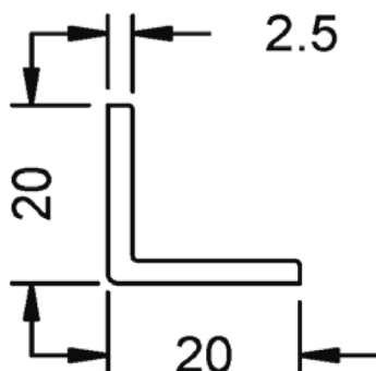
18781 - Profilo angolare da 20/20/2,5 mm.
