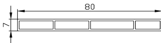
67S80 - Profilo scatolato senza biadesivo 80/7
