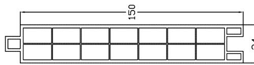
Profilo doga cassonetto
