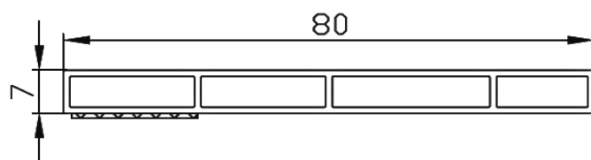
67080 - Profilo scatolato con biadesivo 80/7
