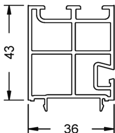
18029 - Adattatore guida avvolgibile 43/36 per 19151
