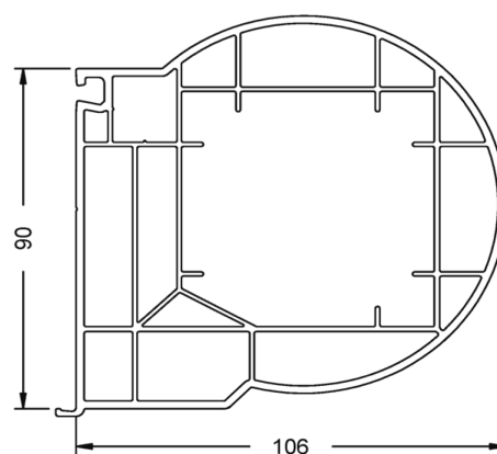
19831 - Profilo di accoppiamento angolo variabile Classic 70 e Living 82
