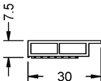
17710 - Profilo scatolato con biadesivo 30/7,5
