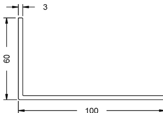
18399 - Profilo angolare da 100/60/3 mm.
