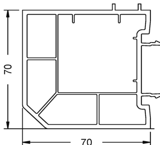
18579 - Profilo di accoppiamento 70 mm Angolo 90° Classic 70
