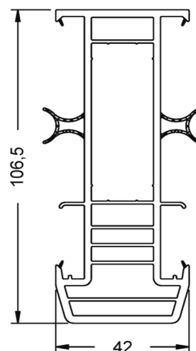
19212- Profilo Lesena 106,5/42 Living 82
