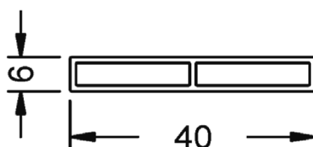
171171 - Profilo scatolato senza biadesivo 40/6
