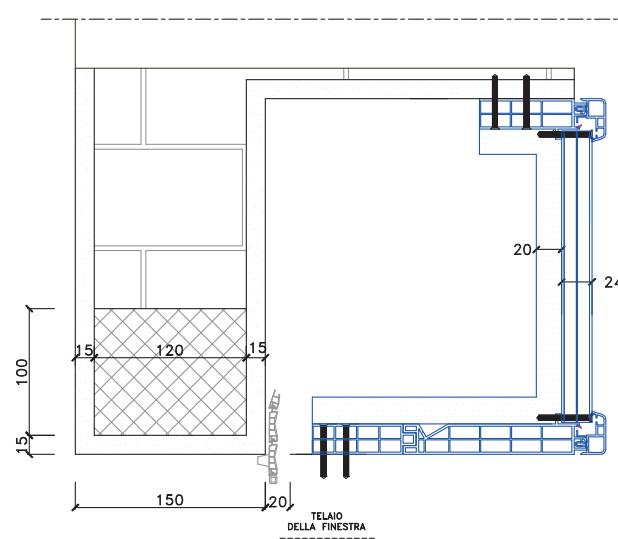
Versione da 24 mm. con isolante termico da 20 mm
