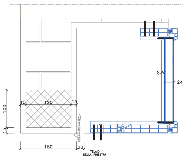
Versione da 24 mm. con isolante termico da 8 mm
