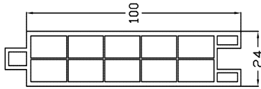
Profilo doga cassonetto
