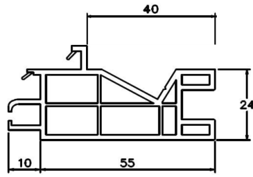
Profilo principale cassonetto ridotto
