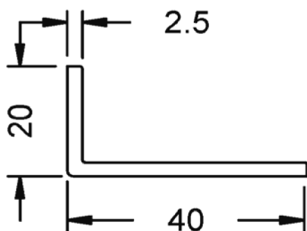
19307 - Profilo angolare da 40/20/2,5 mm.
