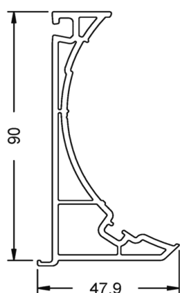
19830 - Profilo di accoppiamento angolo variabile Classic 70 e Living 82
