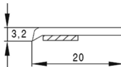
67020 - Piatta con biadesivo da 20 x 3 mm.
