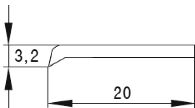
67S20 - Piatta senza biadesivo da 20 x 3 mm.
