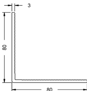
18475 - Profilo angolare da 80/80/3 mm.
