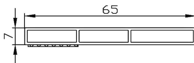
67065 - Profilo scatolato con biadesivo 65/7
