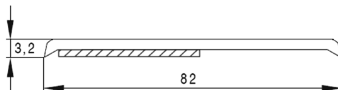
67082 - Piatta con biadesivo da 82 x 3 mm.
