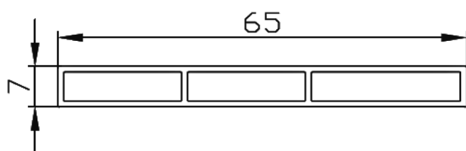
67S65 - Profilo scatolato senza biadesivo 65/7
