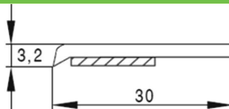
67030 - Piatta con biadesivo da 30 x 3 mm.
