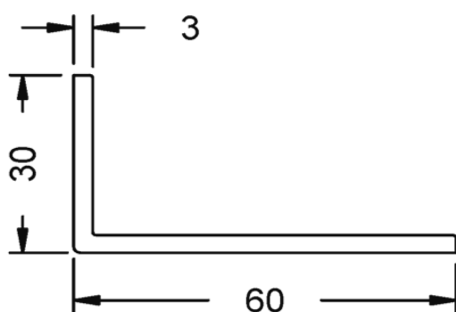
18398 - Profilo angolare da 60/30/3 mm.
