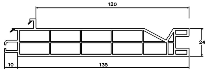
Profilo principale cassonetto standard
