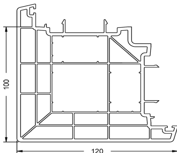
18485 - Profilo di accoppiamento 120 mm Angolo 90° Classic 70 e Living 82
