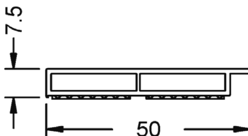
18737 - Profilo scatolato con biadesivo 50/7,5
